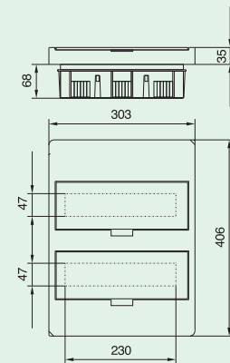
BC-U-2/24(-TW)-ECO
