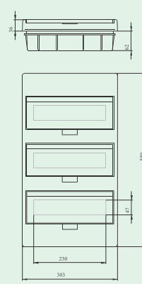
BC-U-3/36(-TW)-ECO
