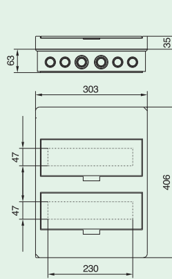
BC-0-2/24(-TW)-ECO
