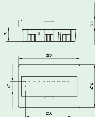
BC-U-1/12(-TW)-ECO
