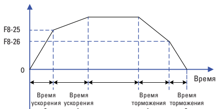
Выходная частота
