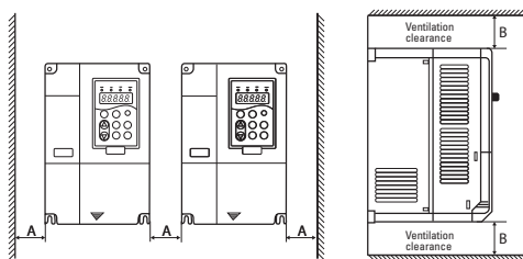
Монтажная схема верхнего и нижнего устройства
