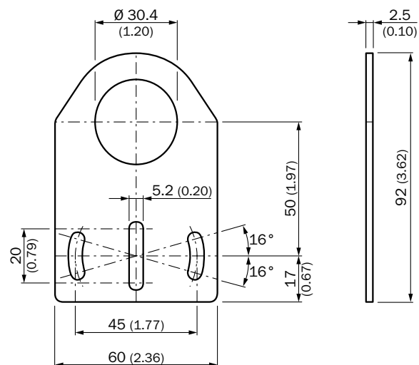
BEF-W4-A
