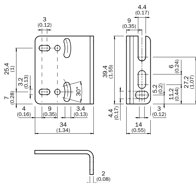
BEF-W4-A
