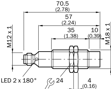
IN30-E0305K
