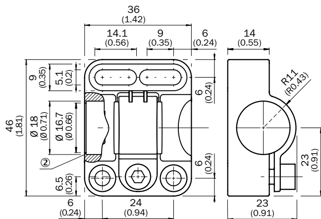
BEF-KHF-M18
