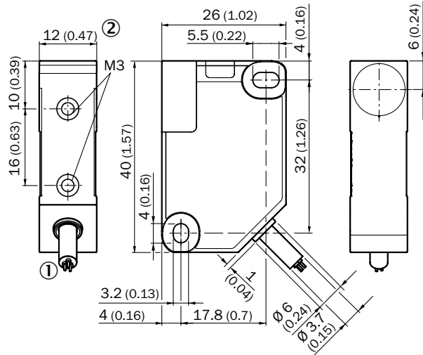
IQ12, cable
