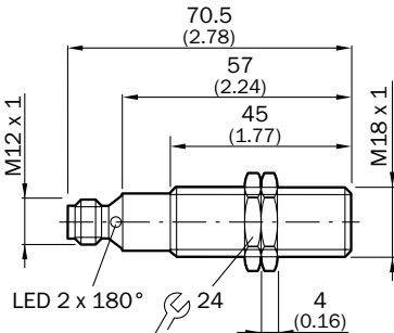
IN30-E0306K
