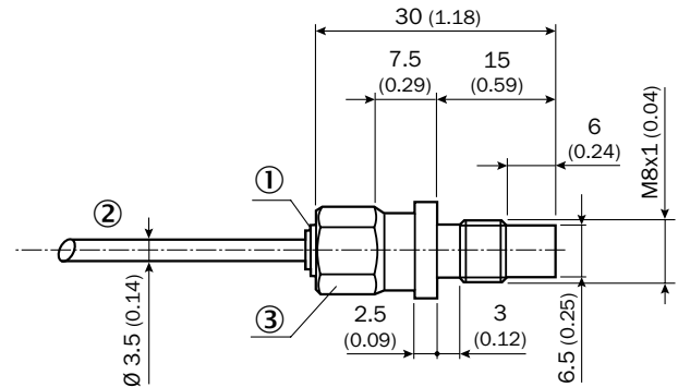
IMP08
