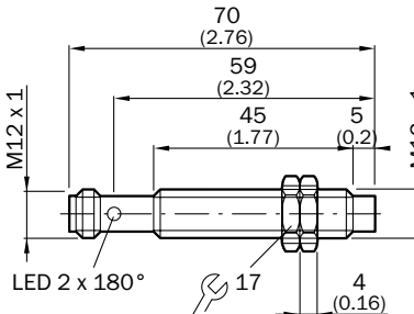
IN30-E0407K
