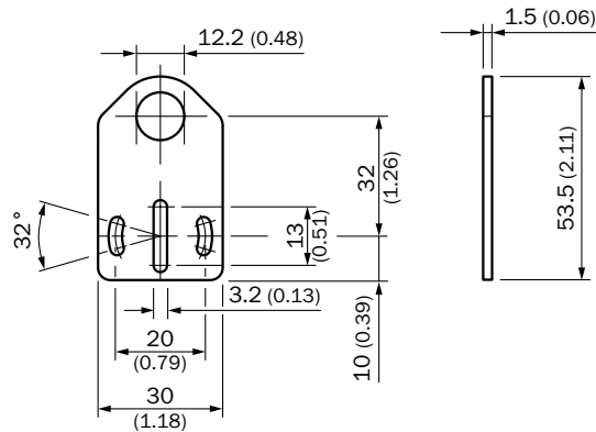
BEF-WG-M12 / BEF-WG-M12N
