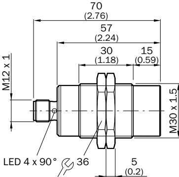
IN30-E0208K
