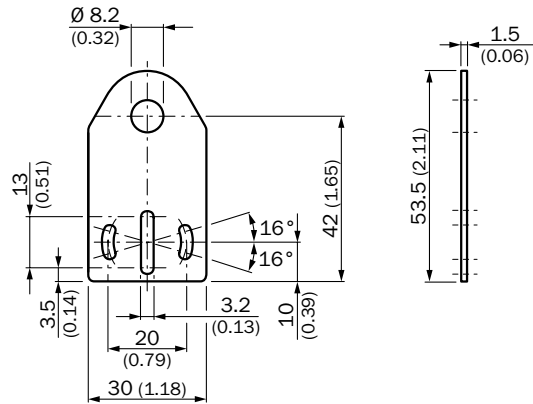
BEF-WG-M08
