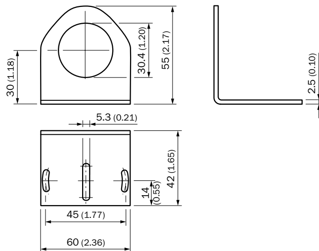
BEF-W4-B
