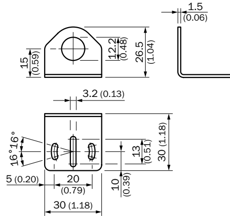
BEF-WN-M18 / BEF-WN-M18N
