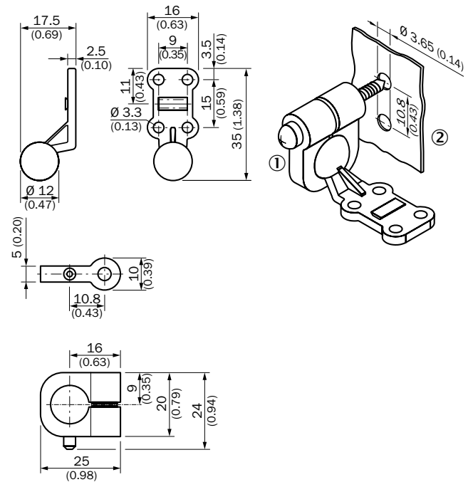
BEF-KH-M08
