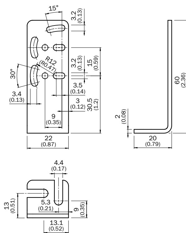
BEF-W4-B
