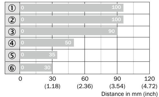
MMxx-90Axx-xxx
