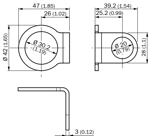
BEF-KHS-N10 / BEF-KHS-N10N
