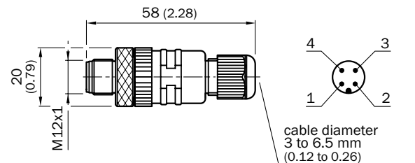
STE-1204-TN
