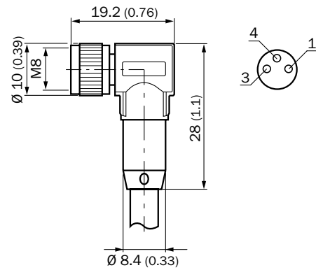
DOL-0803-LxxMC
