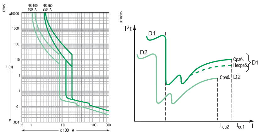
Время-токовые характеристики и кривые энергии аппаратов Compact NSX 100 и 250 А.
