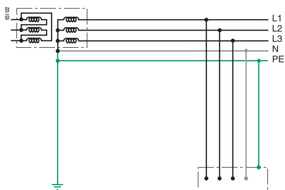
Система TN
