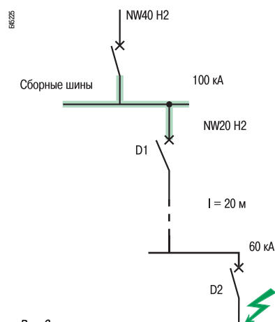
Рис. 2 Полная селективность
