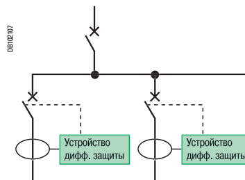
Селективность «по горизонтали»
