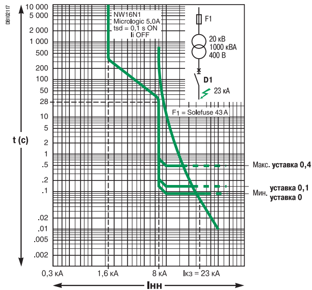
Селективность NW16N1/Solefuse, ток приведен ко вторичной обмотке
