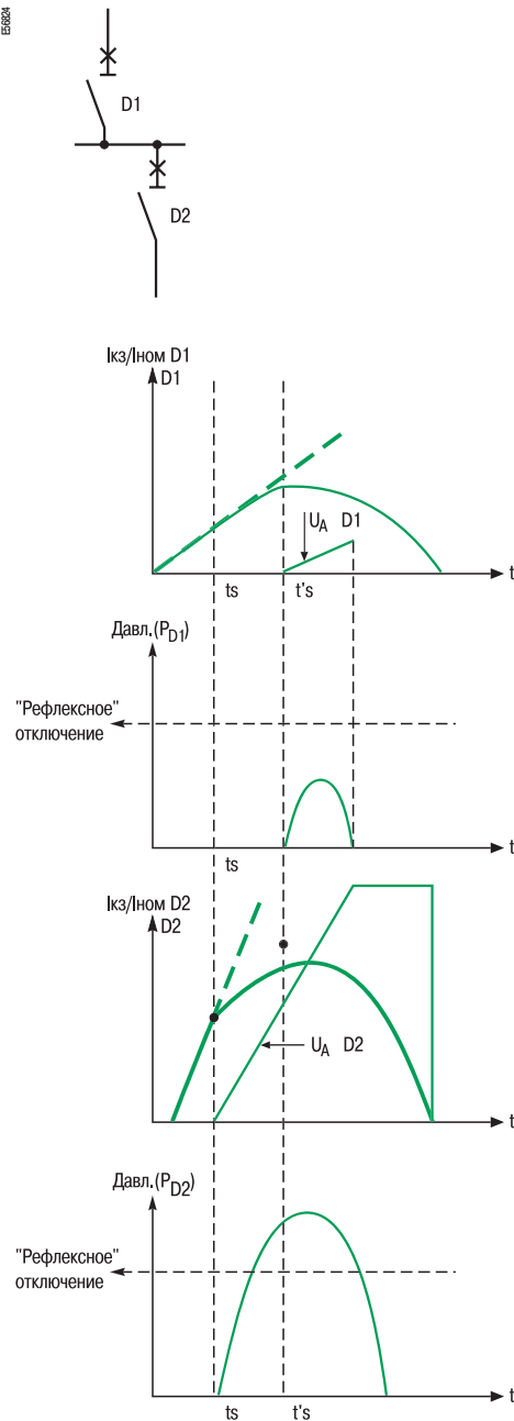
Селективность, усиленная каскадным соединением: описание принципа
