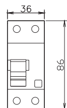
2П RCCB-ID 125 A
