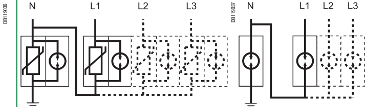
PRD1 25r (1P+N, 3P+N)
