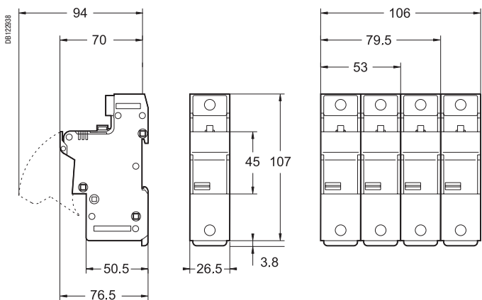
Размеры (мм)
