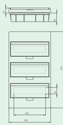
BC-U-3/36(-TW)-ECO
