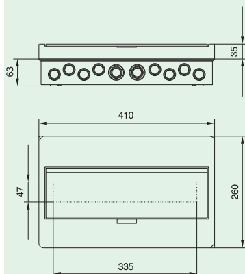
BC-0-1/18(-TW)-ECO
