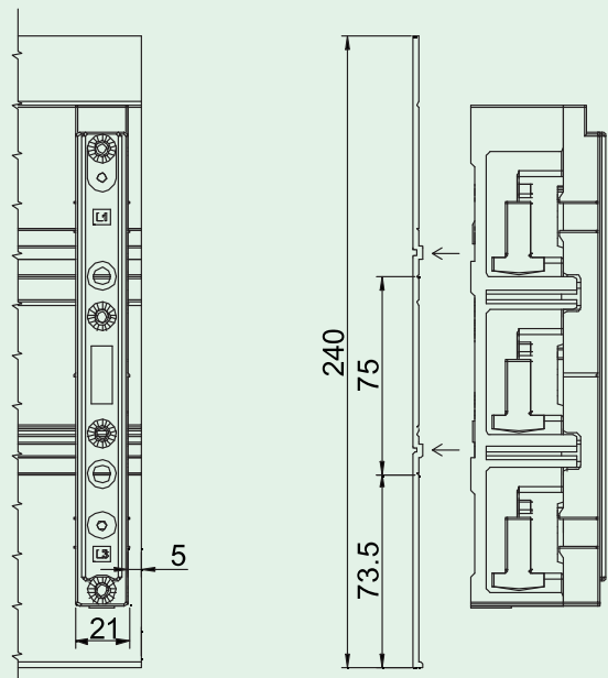
BBS-3/FL-NA
