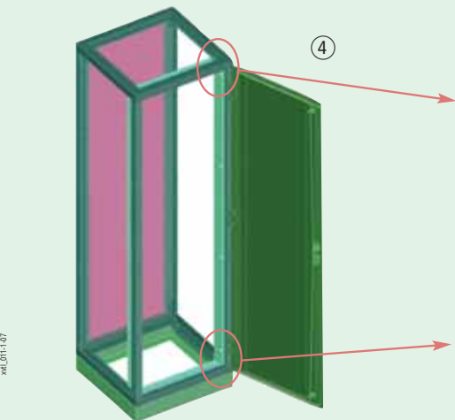
Деталь
