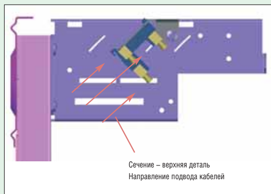
Деталь 2 – сечение
