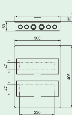
BC-0-2/24(-TW)-ECO
