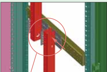
Деталь монтажа XVTL-VP на XVTL-HP/L
