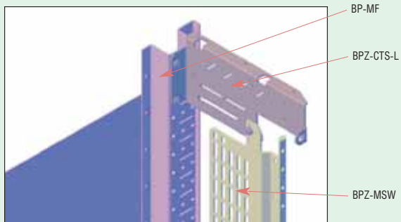
Деталь
