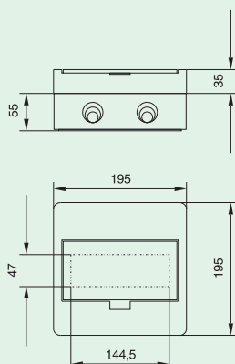
BC-0-1/8(-TW)-ECO
