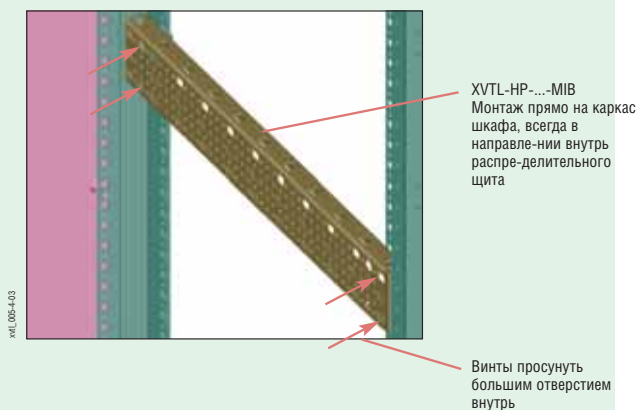
Деталь
