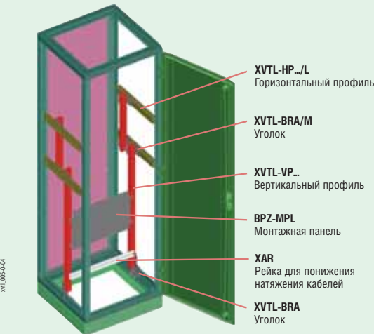
Деталь монтажа XVTL-VP на XVTL-BRA
