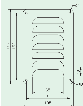
LVP-20V12-CS
