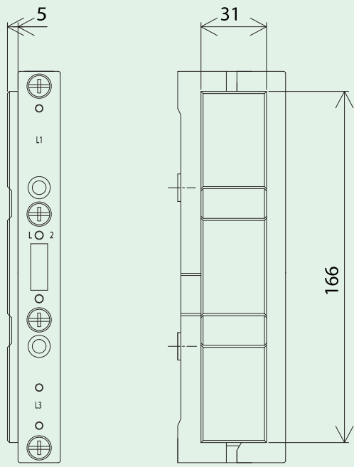
ES-BBS-3/FL
