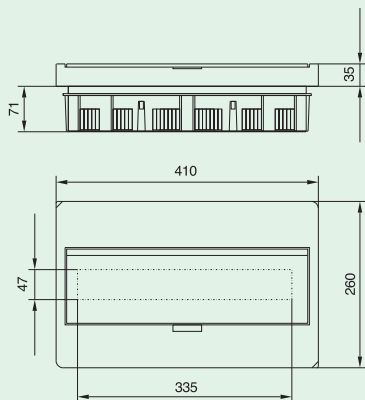
BC-U-1/18(-TW)-ECO
