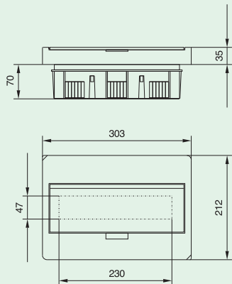
BC-U-1/12(-TW)-ECO
