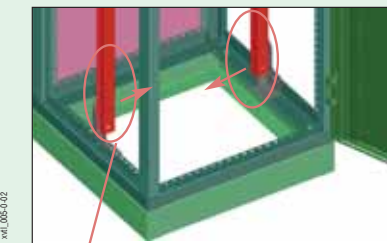
Деталь монтажа XVTL-VP на XVTL-BRA
