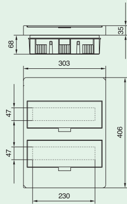
BC-U-2/24(-TW)-ECO
