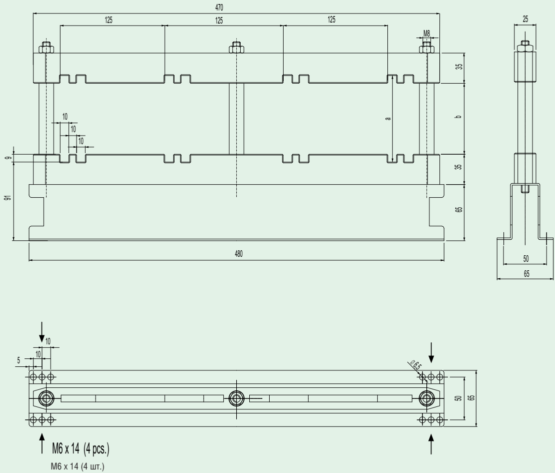
Размеры [мм]
