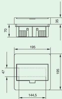
BC-U-1/8(-TW)-ECO
