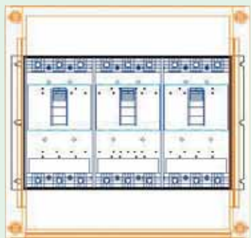
BPZ-NZM3X-...
