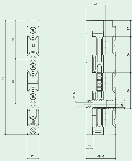
BBS-3/FL
