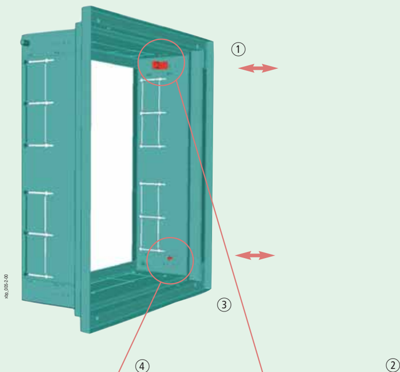
Деталь нижнего ухвата
