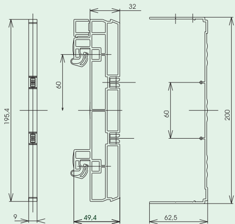
BBC-RCOV1
