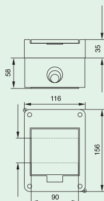
BC-0-1/5(-TW)-ECO
