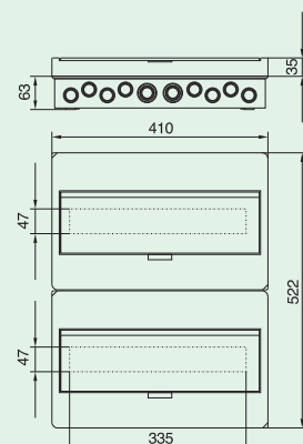
BC-0-2/36(-TW)-ECO
