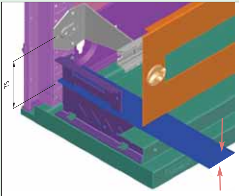
Деталь
