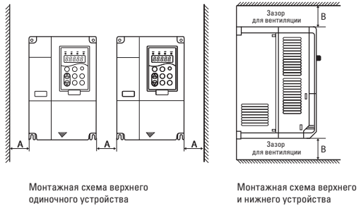
Рис. 4-1 Монтажная схема
