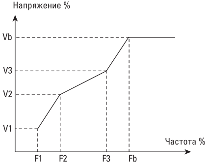
V1-V3: 1-й, 2-й, 3-й проценты частоты многоточечной кривой V/F Vb: номинальный ток двигателя F1-F3: 1-й, 2-й, 3-й проценты частоты многоточечной кривой V/F Fb: номинальная рабочая частота двигателя
