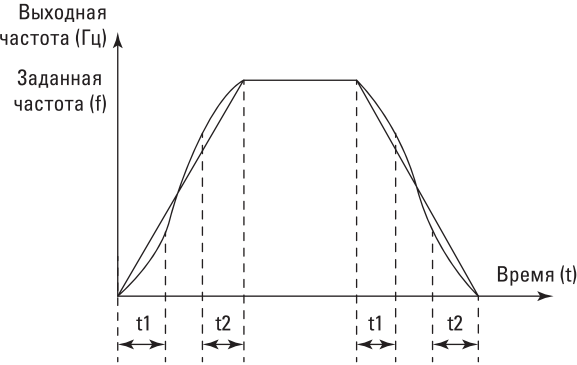
Рис. 6-11 Схема ускорения/замедления А для кривой S
