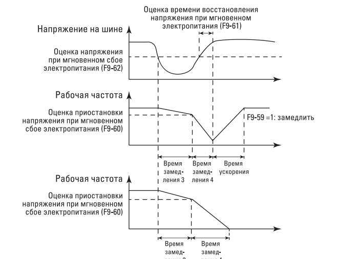
Рис. 6-25. Схема действия при мгновенном сбое электропитания
