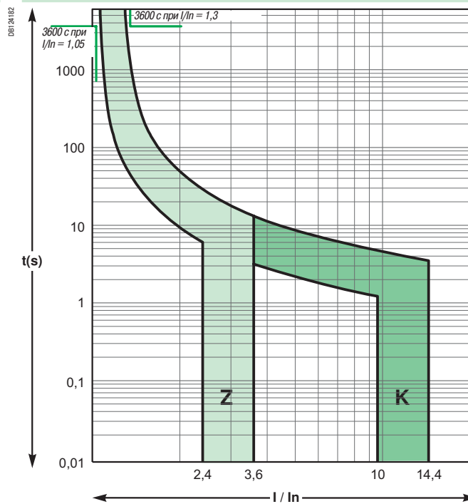
Кривые Z, K, токи до 4А включительно
