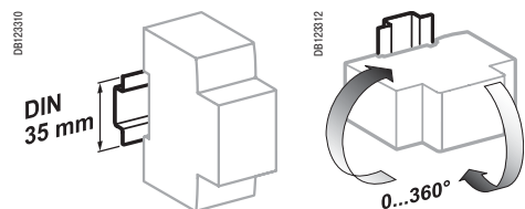
Крепление защёлкиванием на DIN-рейке 35 мм
