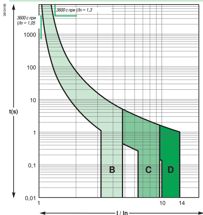
Кривые В, С, D, токи 6-63А включительно
