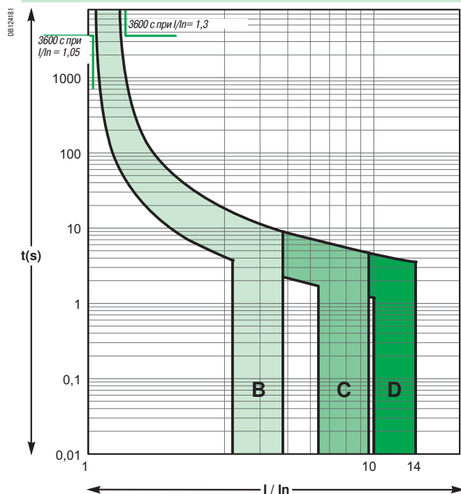
Кривые В, С, D, токи до 4А включительно
