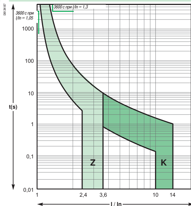
Кривые Z, K, токи 6-63А включительно
