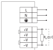
Рис. 1 Схема подключения блока питания
