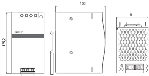
Рис. 3 Габаритные размеры блока питания DR-75W-24, DR-120W-24, DRP-240W-24.
