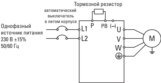
Рисунок 3-2 Стандартное однофазное подключение 0,75–2,2 кВт
