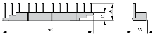
Трехфазные соединители B3.0/4-PKZ4
