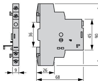
Вспомогательные контакты индикации аварийного срабатывания AGM2...-PKZ... AGM2...-PKZ0
