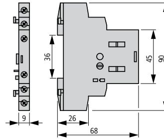
Стандартные вспомогательные контакты NHI...-PKZ... NHI...-PKZ0
